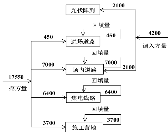
图2-4 土石方平衡图 (m 3 )
