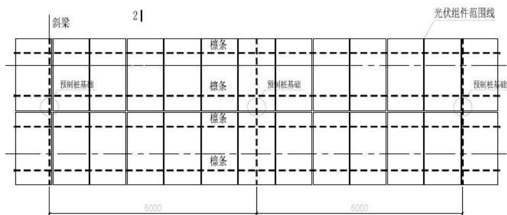
图 2-1 组件平面布置图
